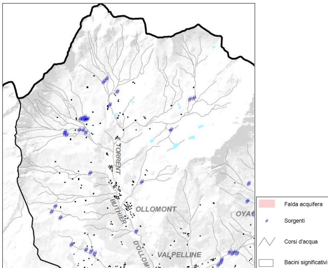
Figura 4.2: carta delle sorgenti
